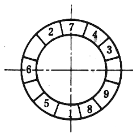
图 F.0.1 吊焊焊缝的试样切取部位示意图
