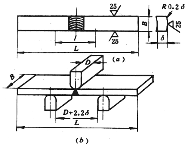
图 F.0.3 冷弯试样规格
