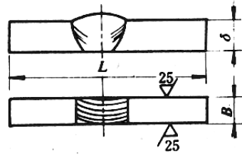
图 F.0.4 金相试样规格
