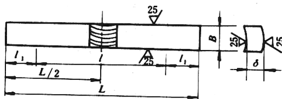
图 F.0.2 拉力试样规格
