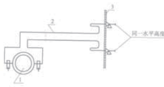
图 3.2.8-3 微差流量测管的安装 1—微差流量测管;2—测量管;3—冷箱壁面
